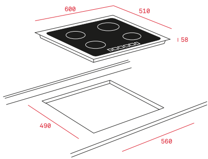
Gerätemaße in mm Breite 600 Tiefe 510 Höhe 58
