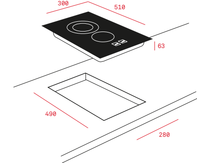
Gerätemaße in mm Höhe 55 Breite 300 Tiefe 510
