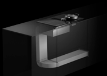
Σωλήνωση για ανακύκλωση με γωνία 90° (έξοδος πίσω)
