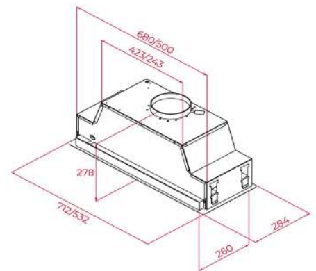
GFL 57651 EOS BK
