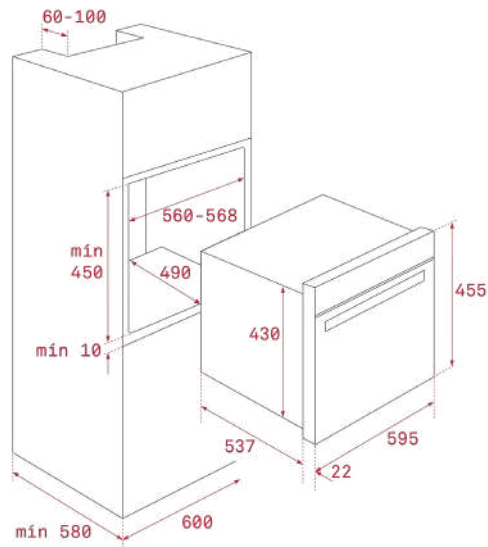
HLC 844 C · MLC 844 · MLC 8440 · MSC 642
