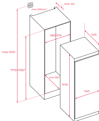
RSF 71725 FI ME / RSL 71735 FI M
