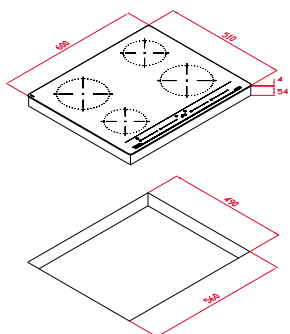
IZC 64010 BK MSS
