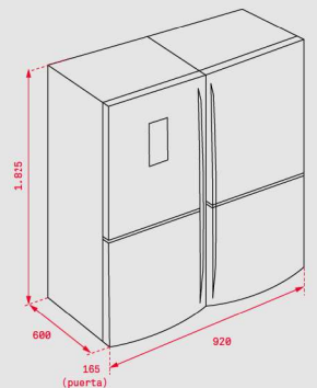
NFE 900 X
