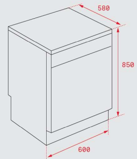
LP8 - 820 BLANCO
