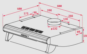
C 6310 INOX.
