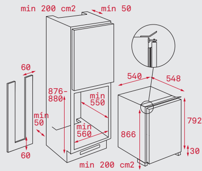
ARTIC TKI3 130 · TKI3 150
