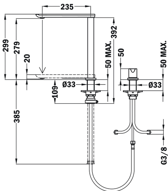
Zwenkbare water uitloop
