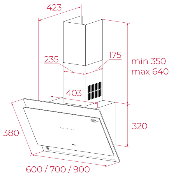
Obvodové odsávanie
