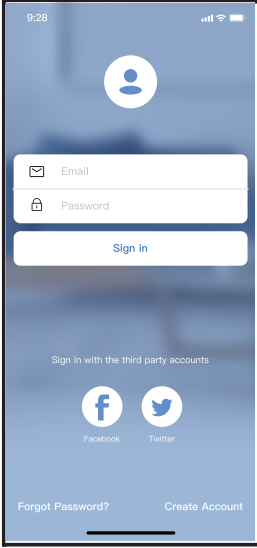
Android
